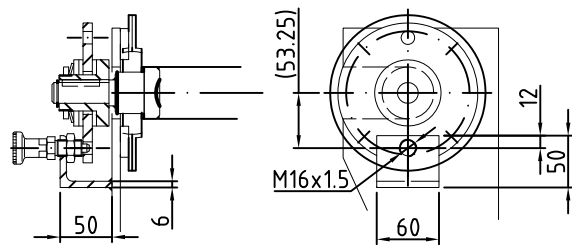
Detail Abrollbremse M. 1:5
