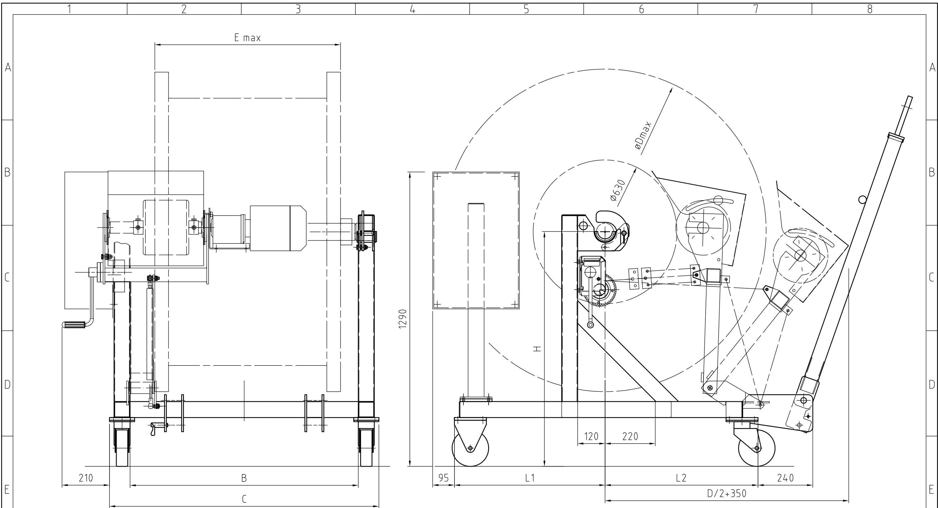
KTA dargestellt mit Trommelantrieb KTA shown with drum drive
